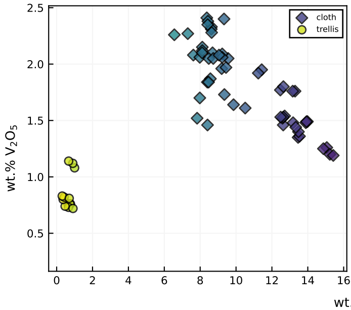
Magnetite
