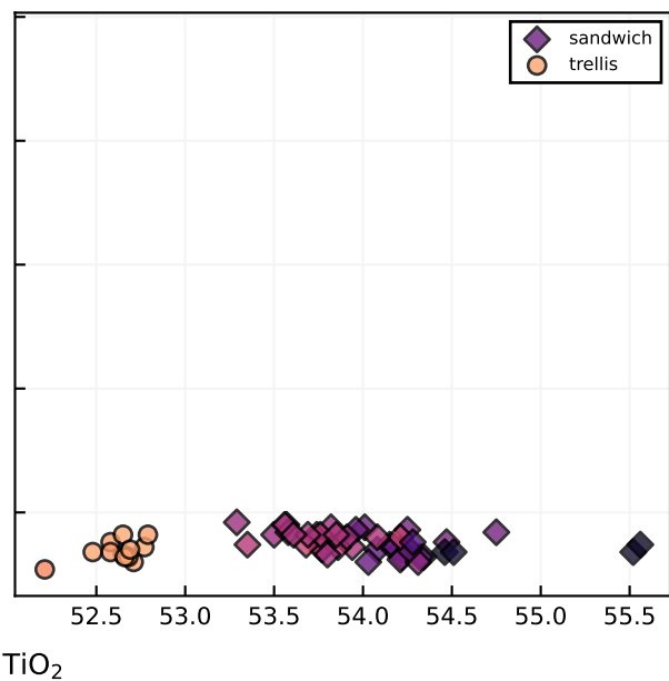
Ilmenite
