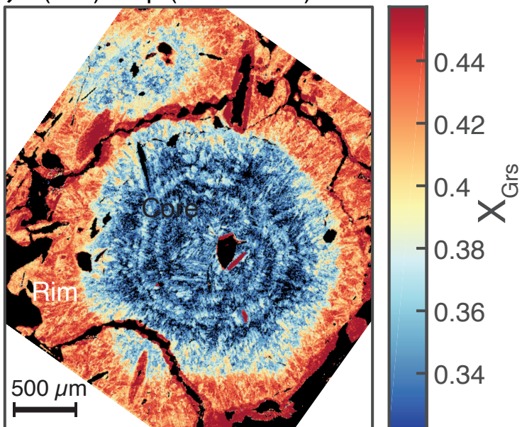
(e) X(Grs) map (Z17TB04B)
