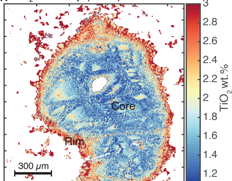
(f) \text{TiO}_2 wt% map (ZTUv)
