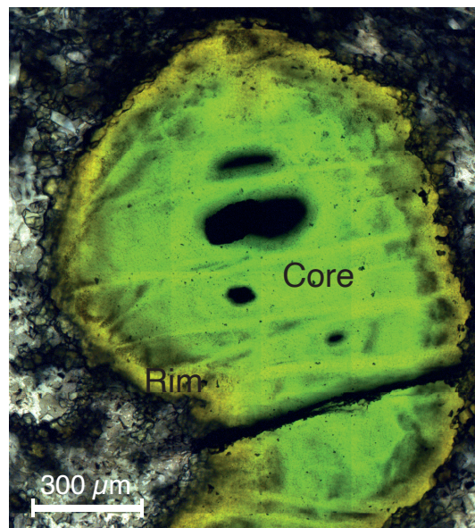
(d) OH content map (ZTUv)
