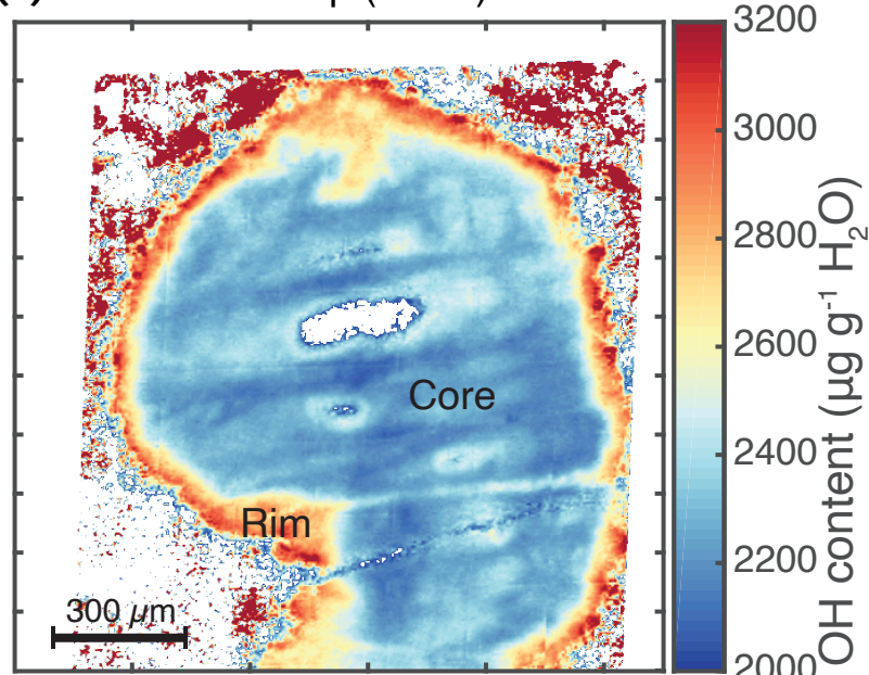
(d) OH content map (ZTUv)
