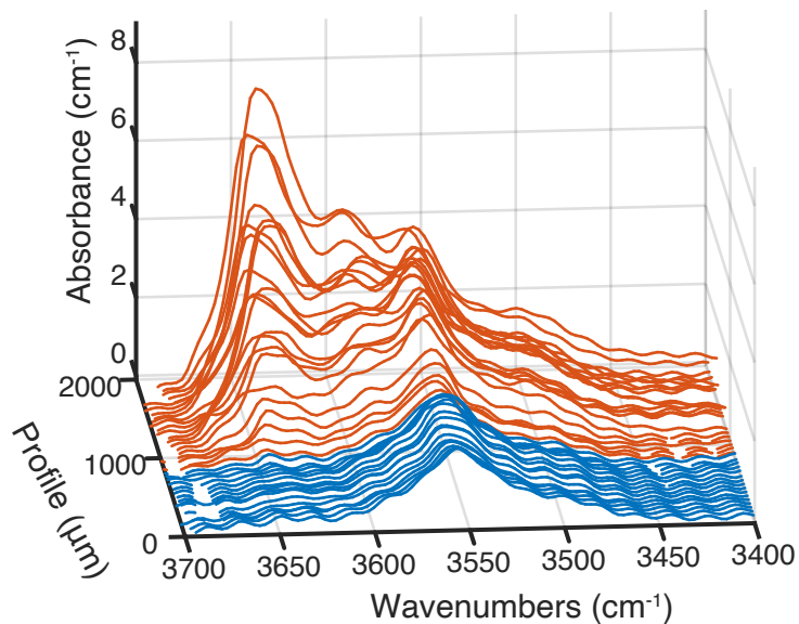
(d) FTIR spectra profile
